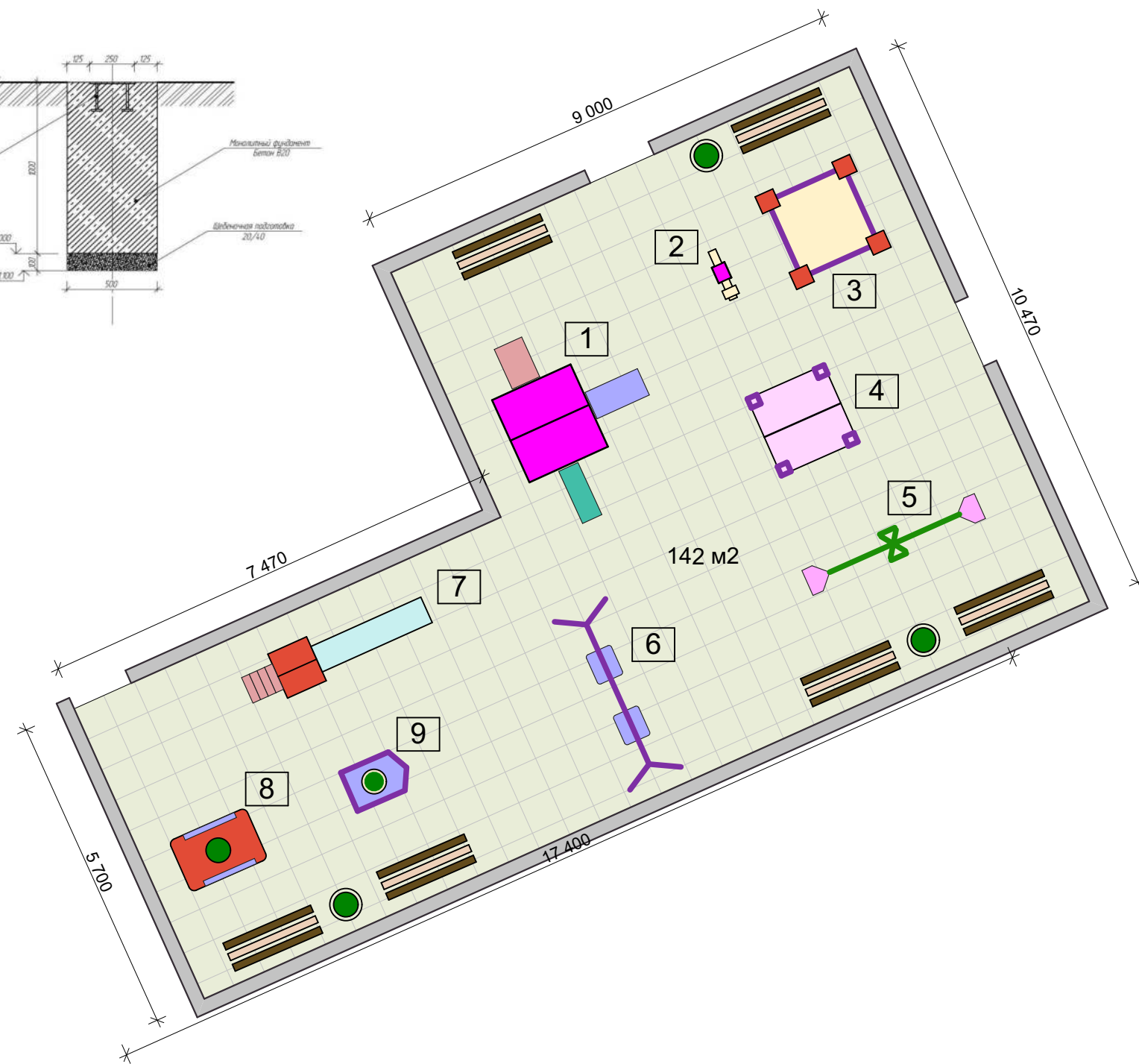
5 Балансир 1480 - 1 шт.
