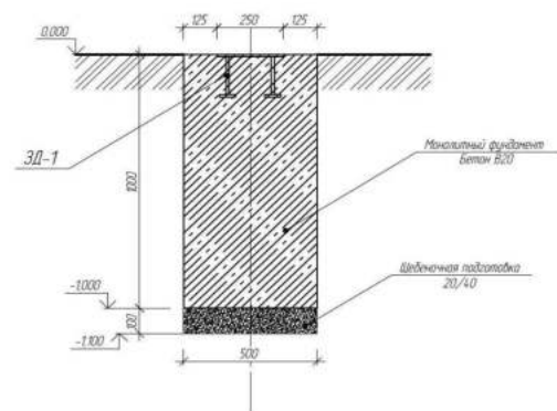
Закладная деталь ЗД-1 для установки оборудования детской площадки
